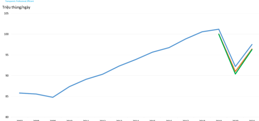
NHU CẦU DẦU THÔ TOÀN CẦU
